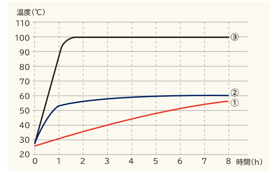
温度特性 ※テスト条件 気温25°C 水温25°C ペール缶内水20ℓ
